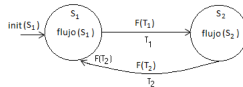
Figura 1. Modelo del autómata híbrido
