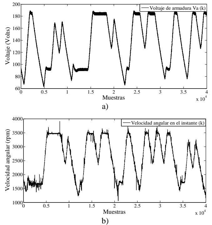
Figura 11. Datos frescos usados en la validación del ANFIS. a) Voltaje de armadura V_a(k) y b) Velocidad angular \omega(k) .
