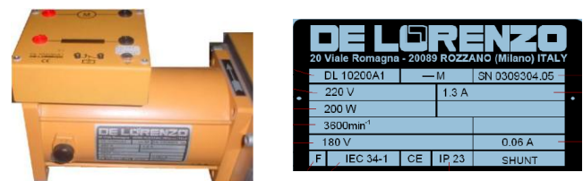
Figura 1. Motor DL10200A1 de la marca De Lorenzo
