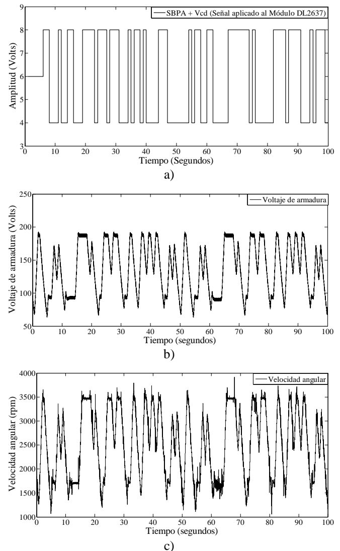
Fig. 6 Forma de la señal de entrada y salida del módulo DL 2637 cuando se le aplica la SBPA, a) SBPA aplicada al módulo DL 2637, b) voltaje aplicado a la armadura del motor y c) velocidad angular del motor.
