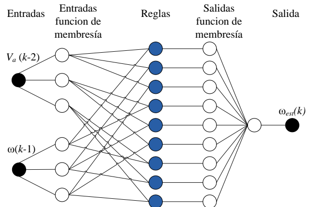
Figura 8 Estructura de la red ANFIS.
