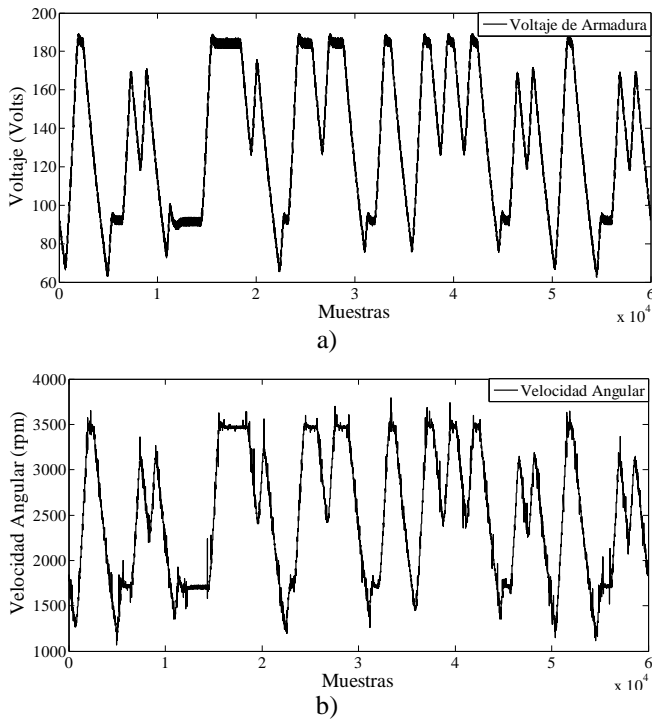
Figura 9 Datos usados en el entrenamiento del ANFIS. a) Voltaje de armadura del motor, b) Velocidad angular del motor.
