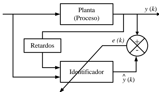
Figura 7. Esquema de Identificación en Serie-Paralelo.
