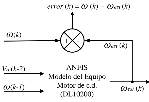
Figura 10 Esquema para Validar el ANFIS por extrapolación.
