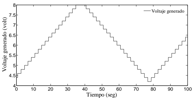
Figura 13 Señal de voltaje aplicada a la fuente variable del módulo DL2637.
