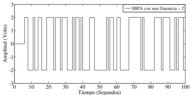
Figura 5. Secuencia binaria pseudoaleatoria generada con el registro de corrimiento de ocho bits.
