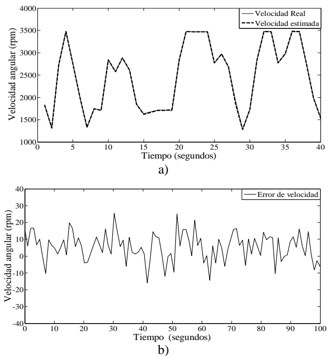
Figura 12 Gráficas para Validar el ANFIS por extrapolación. a) Compara la velocidad real de salida del motor en el instante (k) (-) con la red ANFIS \omega_{est}(k) en el instante (k) , b) Error entre las dos salidas anteriores.
