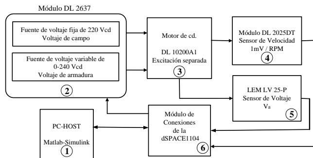
Figura 3 Diagrama de interconexión de los elementos empleados.
