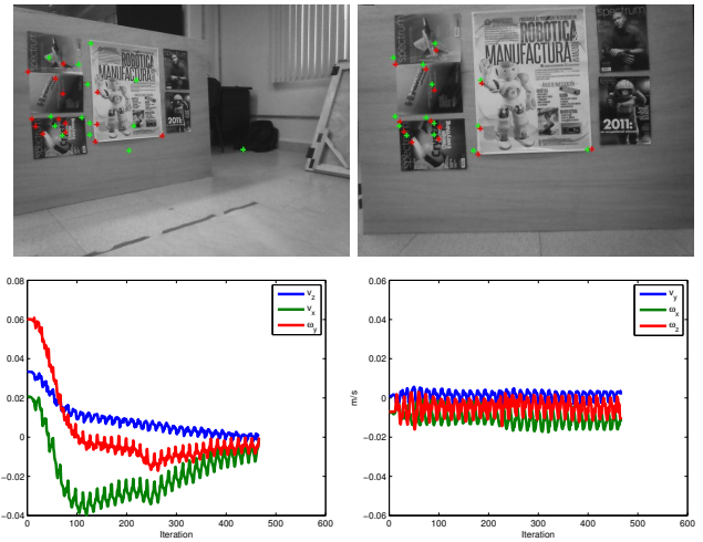
Figura 6. Control 2D con K . Primer renglón: imagen inicial e imagen final. Segundo renglón: velocidades de entrada al GMH y velocidades no requeridas por el GMH.
