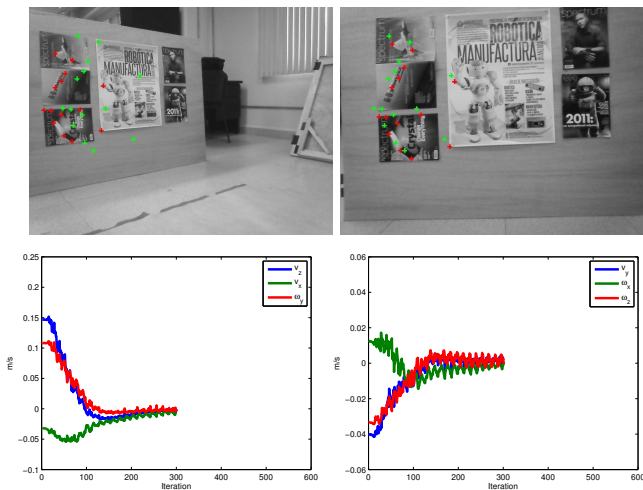
Figura 5. Control 3D con \hat{K} . Primer renglón: imagen inicial e imagen final. Segundo renglón: velocidades de entrada al GMH y velocidades no requeridas por el GMH.
