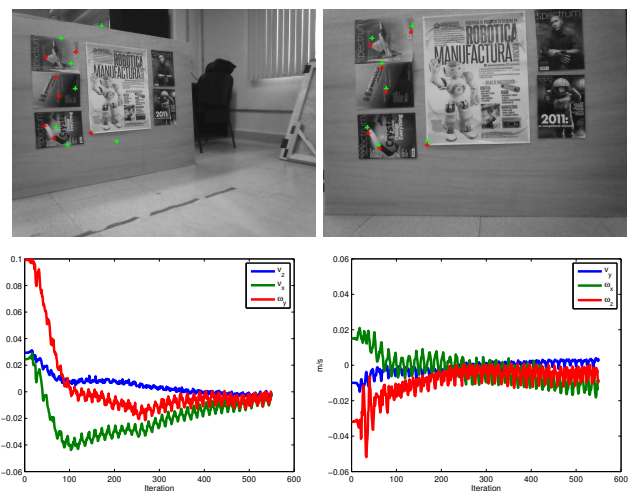
Figura 7. Control 2D con \hat{K} . Primer renglón: imagen inicial e imagen final. Segundo renglón: velocidades de entrada al GMH y velocidades no requeridas por el GMH.
