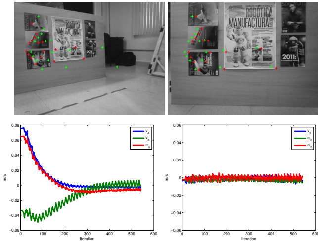
Figura 4. Control 3D con K . Primer renglón: imagen inicial e imagen final. Segundo renglón: velocidades de entrada al GMH y velocidades no requeridas por el GMH.
