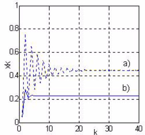
Figura 6. Ciclo de trabajo respecto a la k -ésima iteración. a) a = 0.8 y x^* = 0.44 ; b) a = 0.3 y x^* = 0.23
